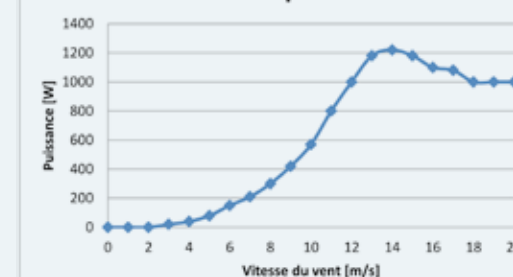
Courbe de puissance
